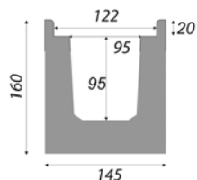
korytka betonowe z pokrywą żeliwną
