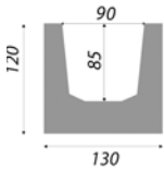
korytka betonowe z pokrywą ocynkowaną
