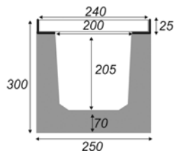
korytka betonowe z pokrywą żeliwną
